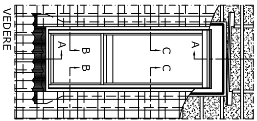
DET. 1 1:5
